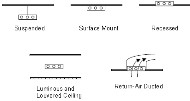
Fig. 1 – Luminaire type
